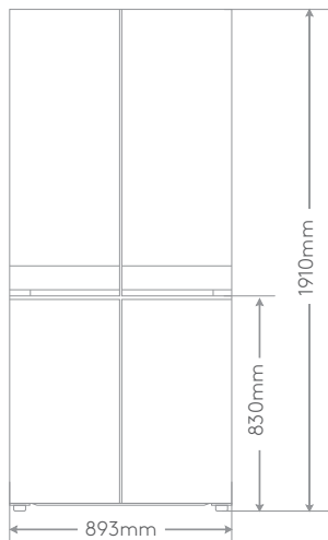
正视图
