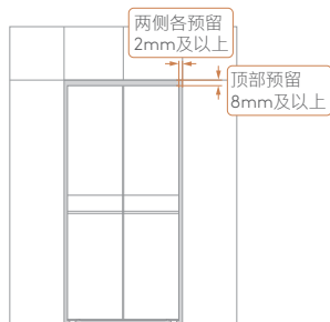
居中安装
