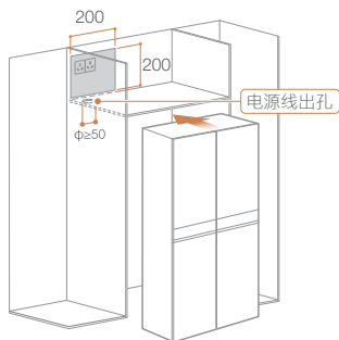
插座位置
